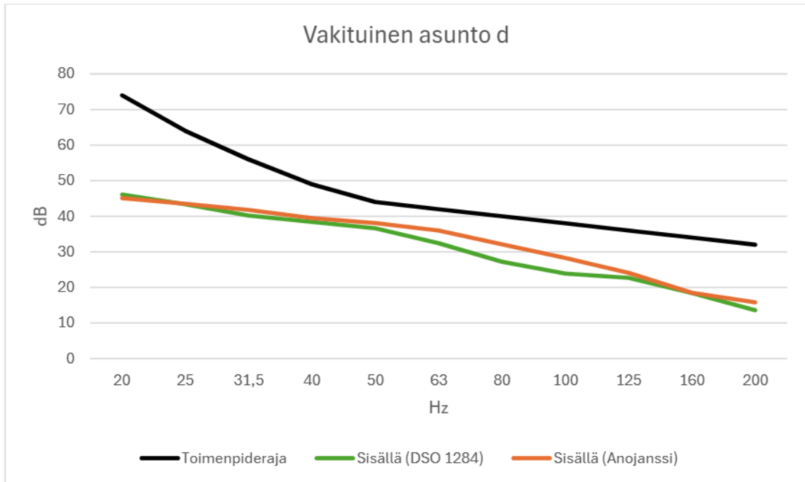
Kuva 3. Ympäristöministeriön ohjeistuksen mukainen pienitaajuisen melun laskenta sekä sosiaali- ja terveysministeriön toimenpiderajat vakituuisessa asunnossa d.
