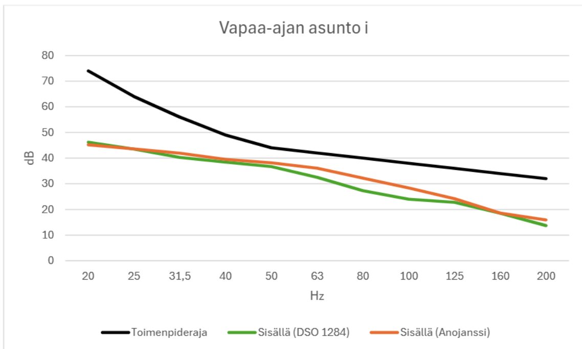
Kuva 2. Ympäristöministeriön ohjeistuksen mukainen pienitaajuisen melun laskenta sekä sosiaali- ja terveystieteiden ministeriön toimenpiderajat vapaa-ajan asunnossa i.
